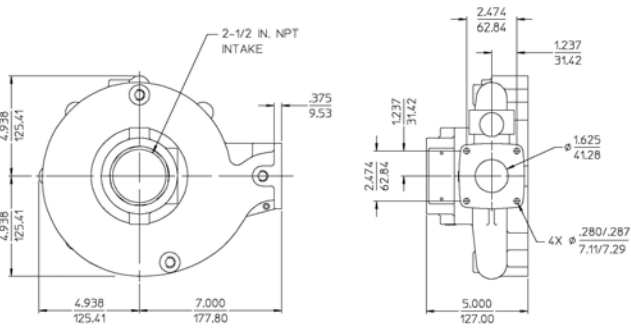
MODEL PB18-2515-LE
