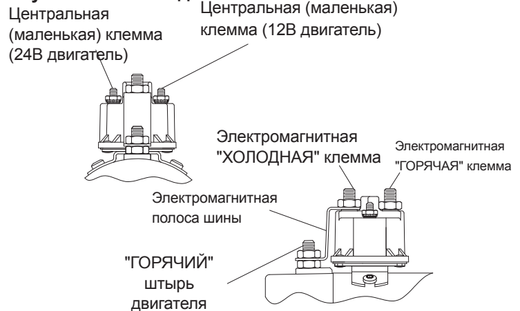
Рисунок 5. Соленоид
