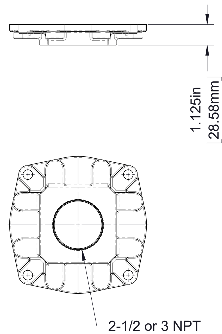
Tapped flange
