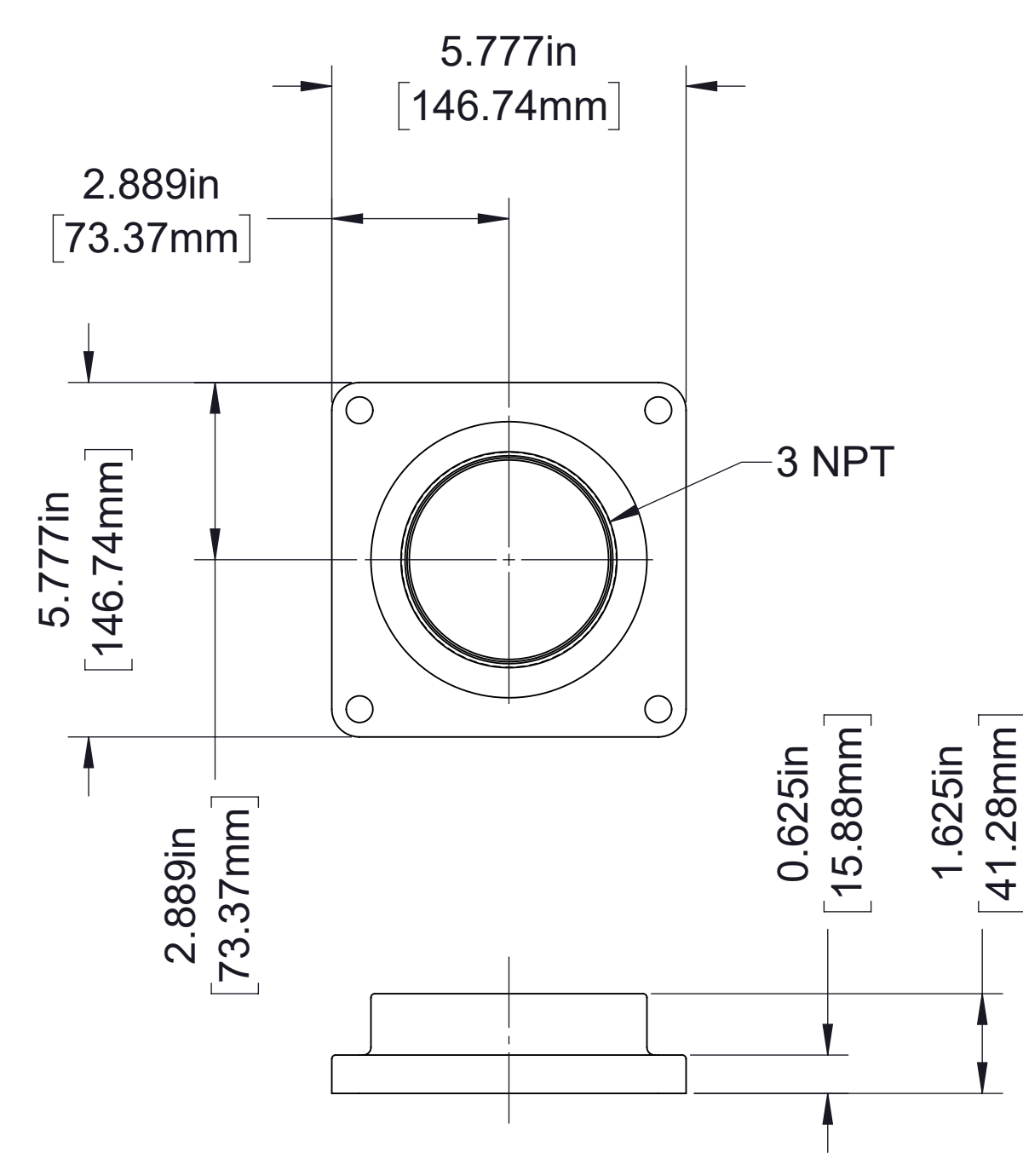
Tapped Flange
