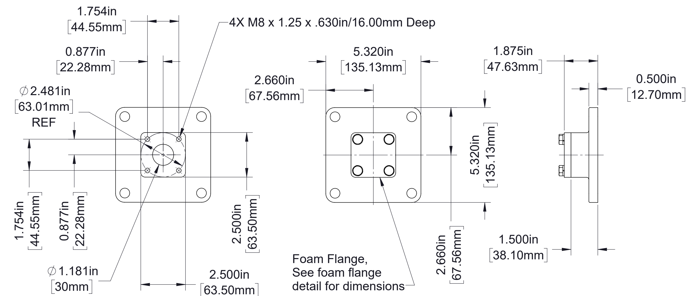
Foam Flange
