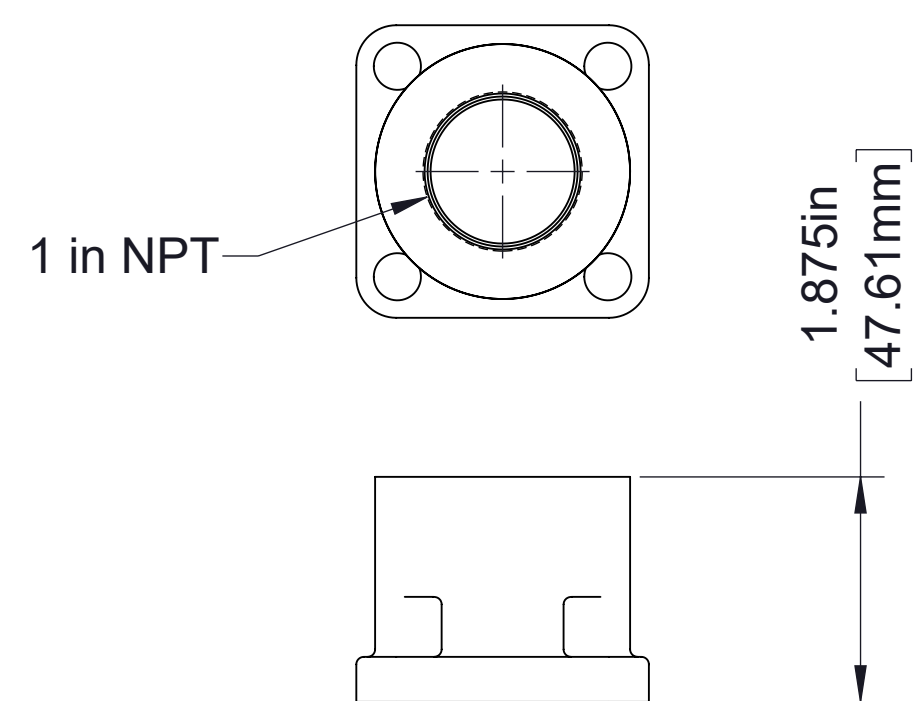
Tapped Flange
