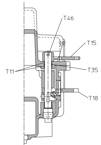
SECTION D-D
