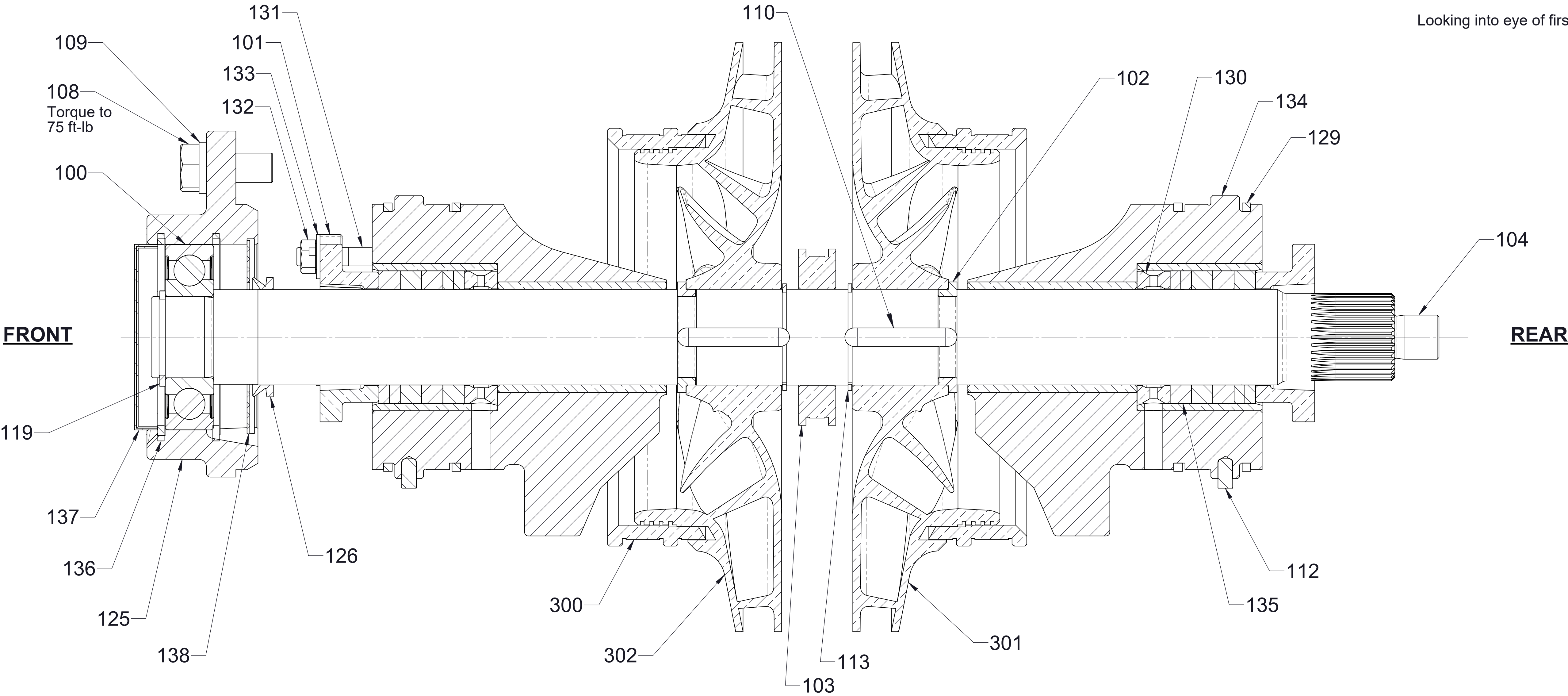
Section A-A
